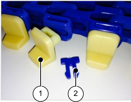
Abb. 3: Montage der Modulbandkette
