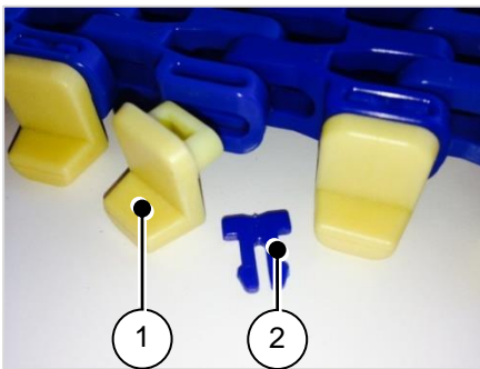
Abb. 4: Modulbandkette anpassen
